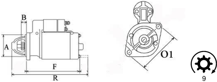
Wymiary:
