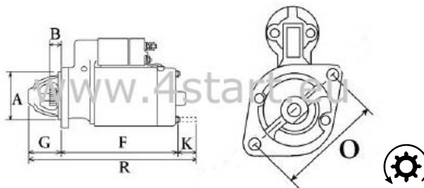
WYMIARY
